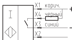
Схема подключения
