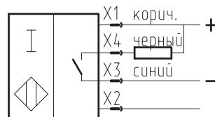
Схема подключения
