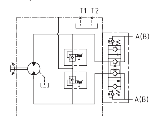
Гидросхема
